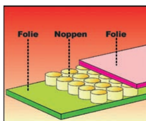
Schichtdarstellung der 3 Lagen
