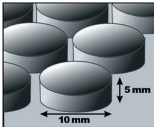
Noppendurchmesser 10 mm Noppenhöhe 5 mm
