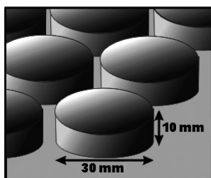
Noppendurchmesser 30 mm Noppenhöhe 10 mm
