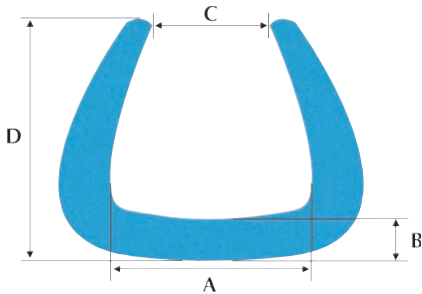
Schaumprofil "Pro U", 9 mm stark, 2 m lang
